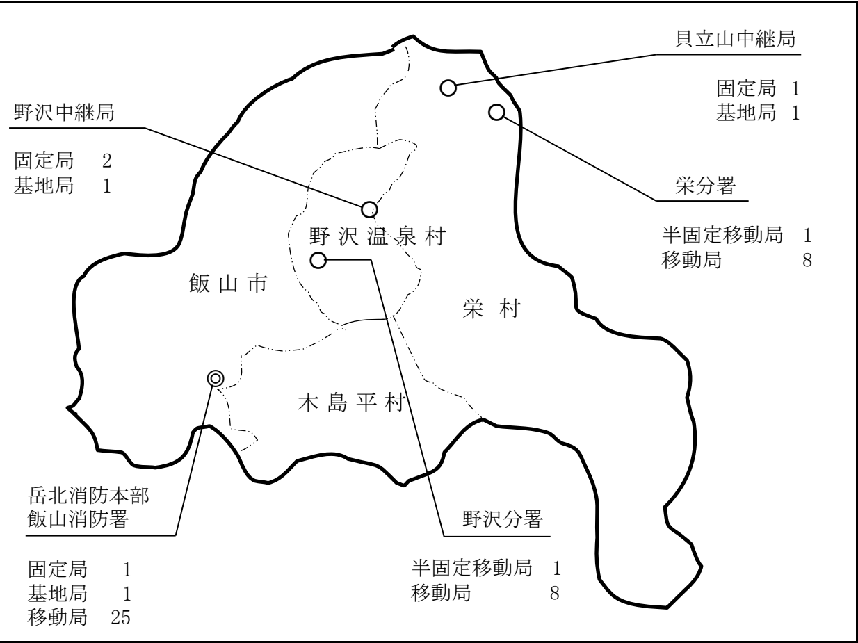
消防通信配置図
