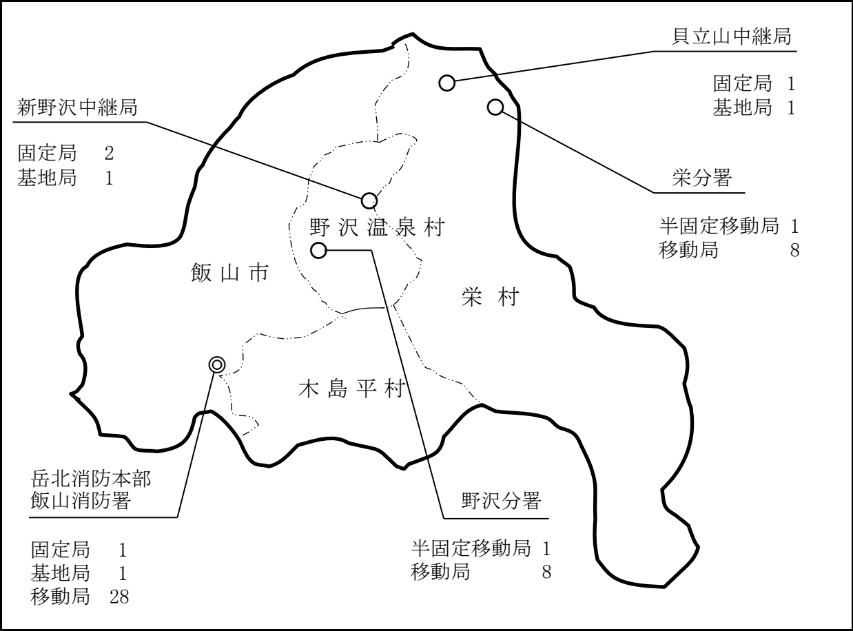
消防通信配置図
